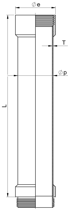
TUBO GETTO / TREMIE PIPE
