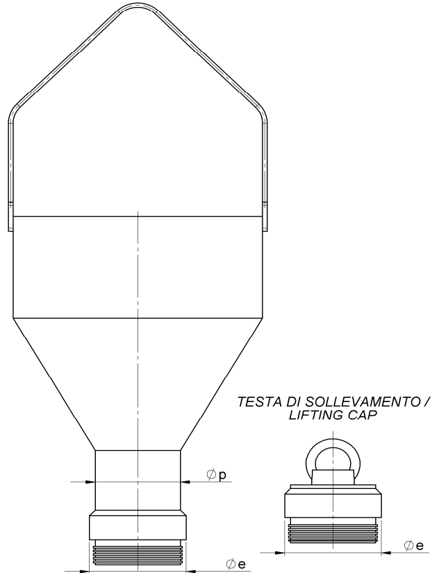
TRAMOGGIA / HOPPER
