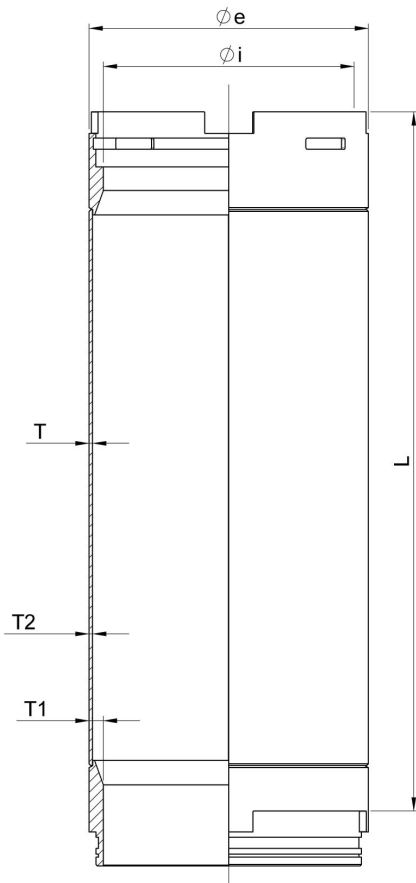
TUBO DI MANOVRA / CASING PIPE
